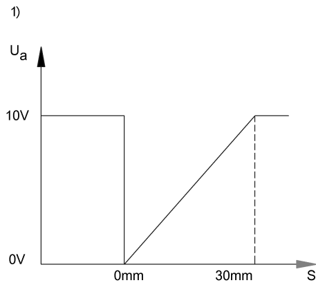
1) Стандартная характеристика
