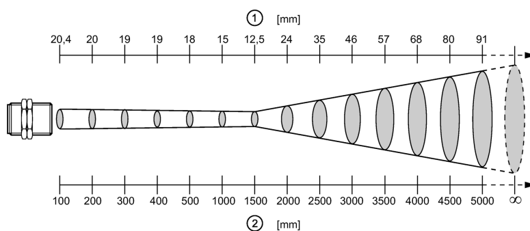
1: Messfleckdurchmesser; 2: Messabstand
