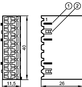
Abbildung zeigt Kontakt-Gehäuse mit geschlossenem Deckel Ansicht auf Kontakt-Einsteckseite
