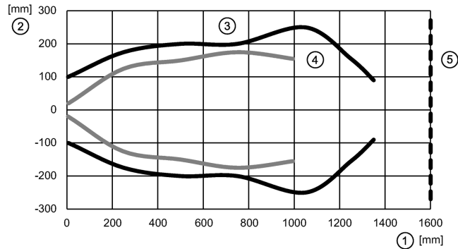
1: Расстояние; 2: Звуковой луч; 3: Мишень 200 x 200 мм; 4: Мишень Ø 25 мм; 5: Отражатель
