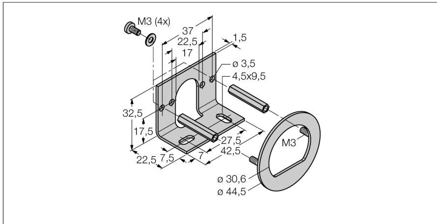
Монтажная рамка и уголок для PK-N с комплектующими
