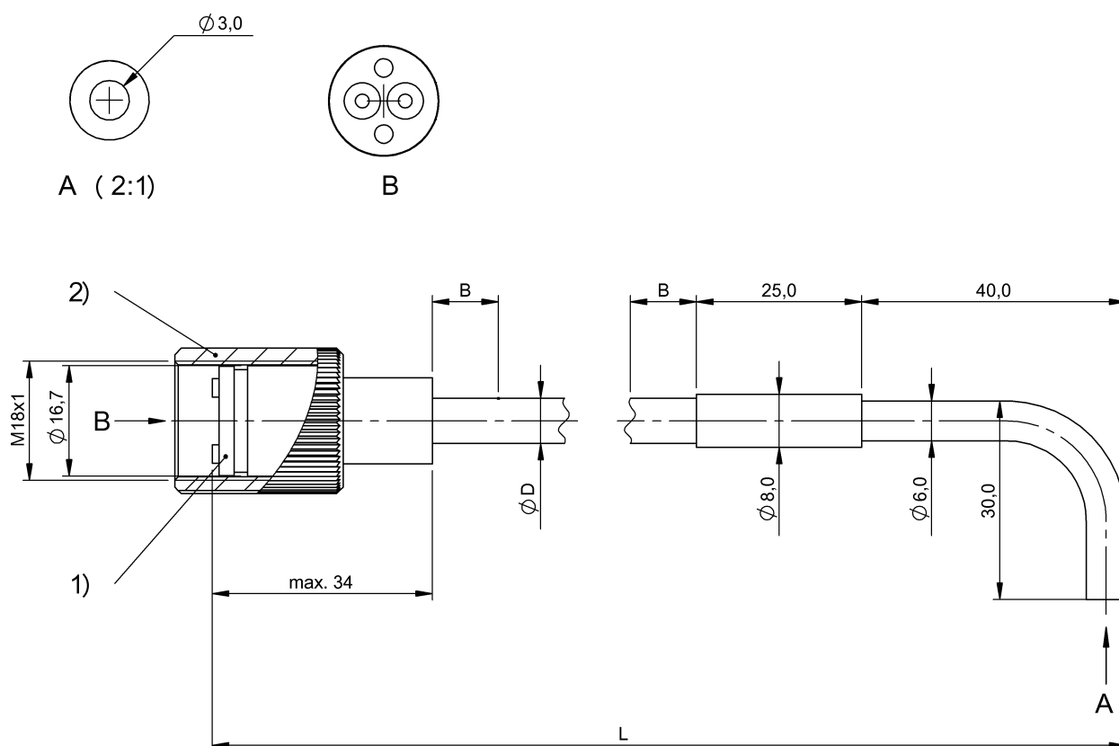
1) Съемная шайба, 2) Накидная гайка
