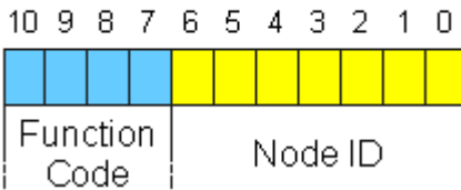
Fig. 139: Default Identifier
