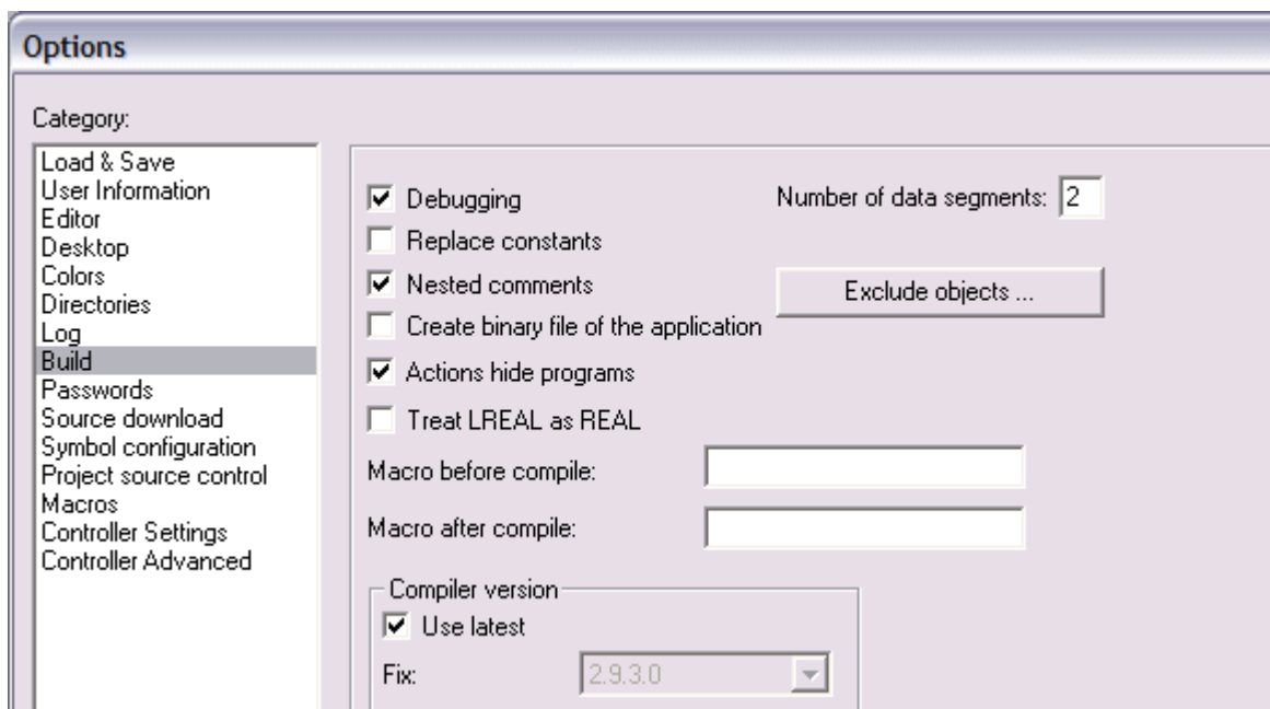
Fig. 81: Build
