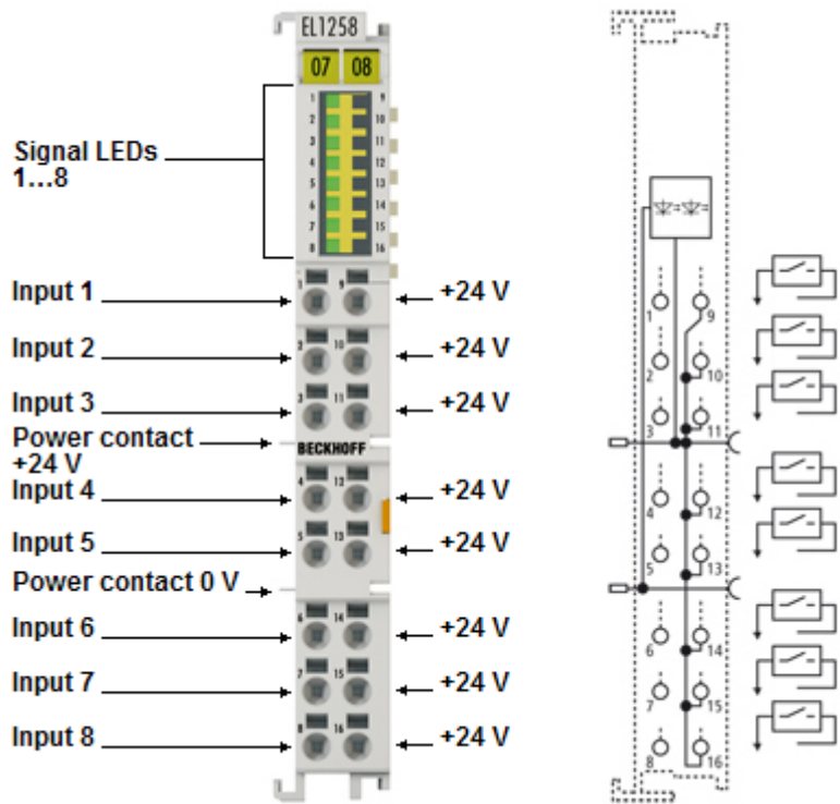
Fig. 39: EL1258
