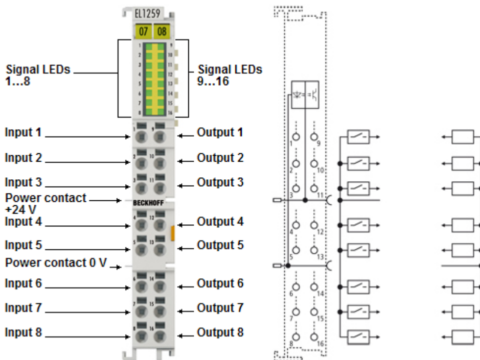
Fig. 10: EL1259
