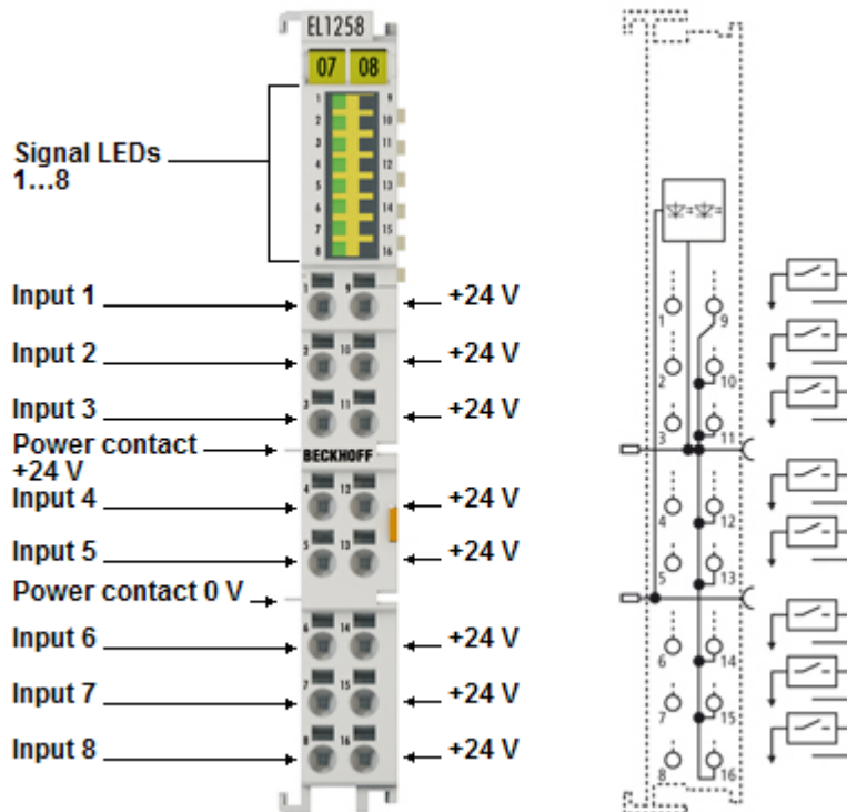
Fig. 9: EL1258
