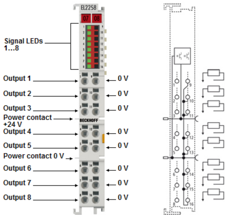
Fig. 41: EL2258
