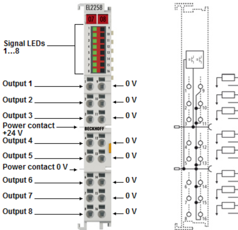
Fig. 11: EL2258
