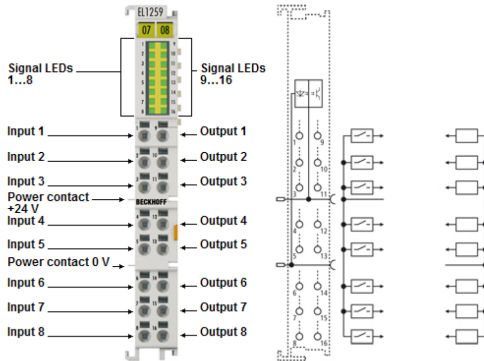
Fig. 40: EL1259
