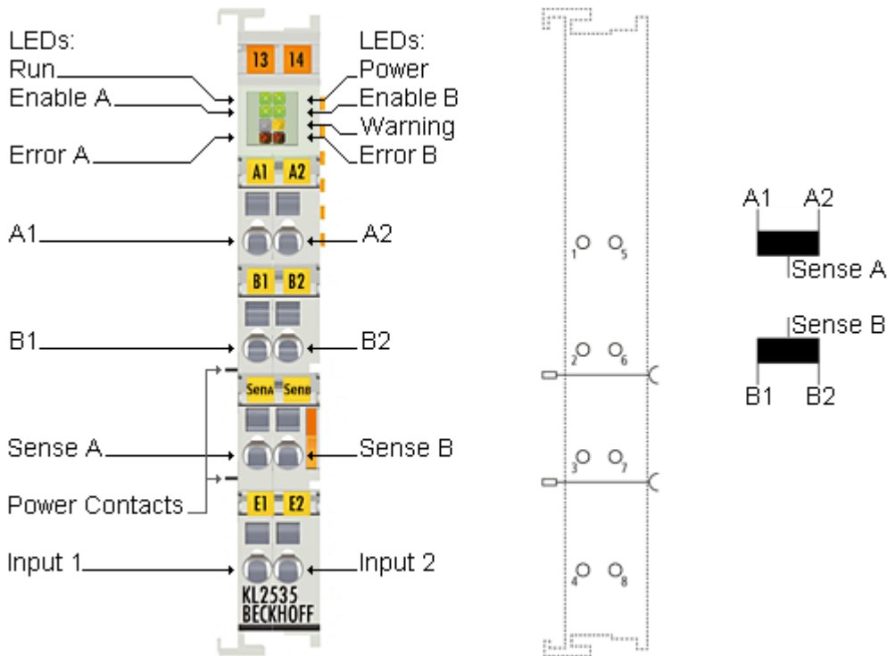
Fig. 2: KL2535 - LEDs
