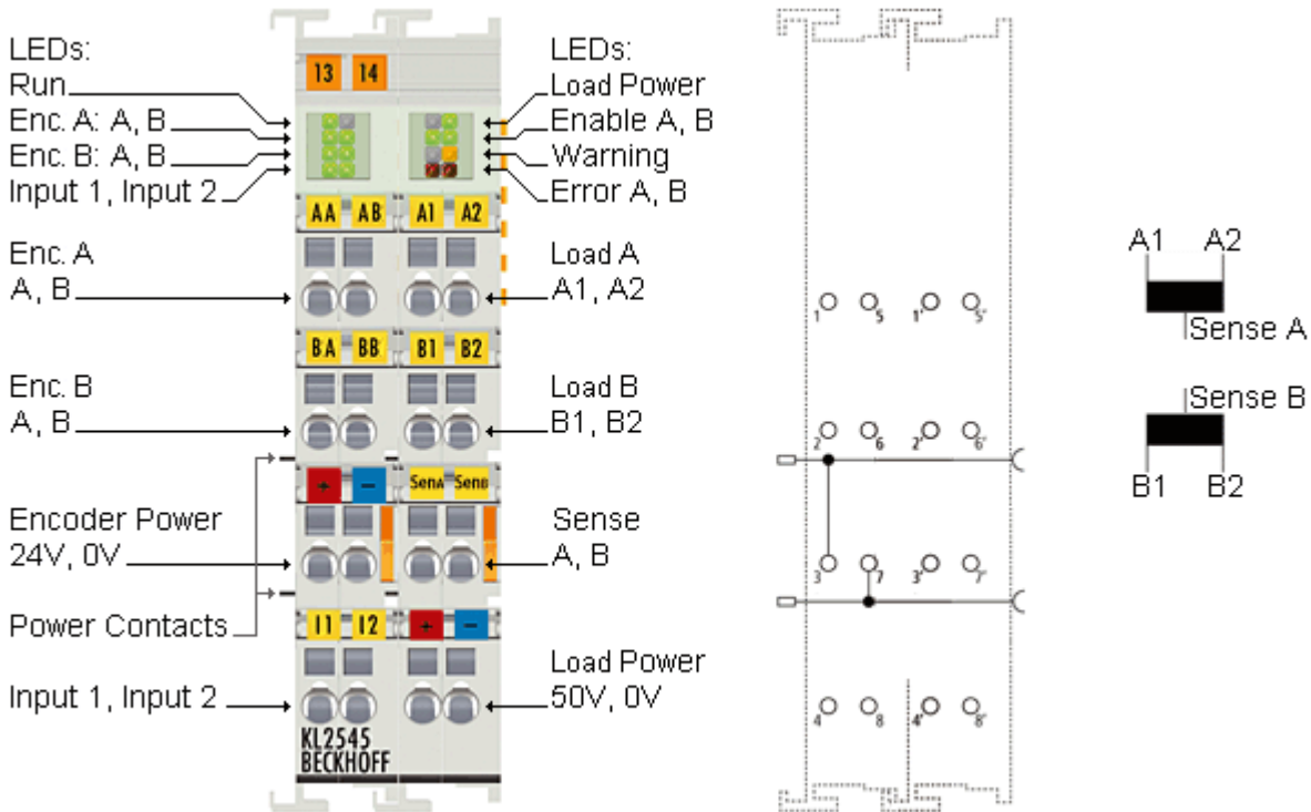
Fig. 4: KL2545 - LEDs
