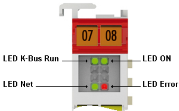
Fig. 4: KL2751, KL2761 - LEDs
