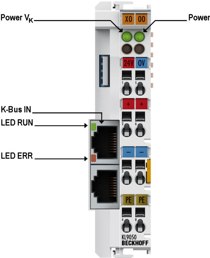
Fig. 15: KL9050 - LEDs
