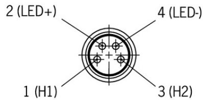
Ansicht auf Steckseite des Lesekopfs
