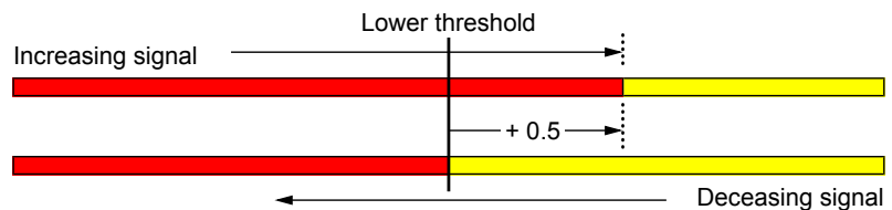
Fig. 90: Hysteresis
