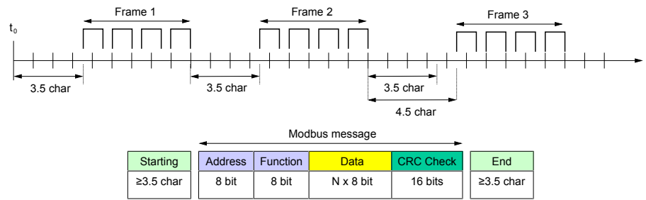
Fig. 102: Modbus Message Frame
