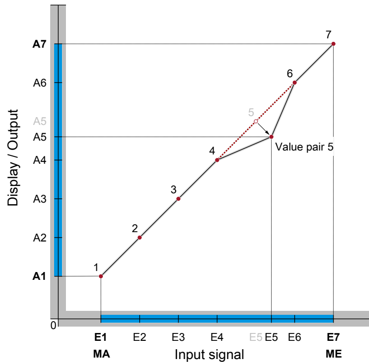
Fig. 73: Table function (n=7)
