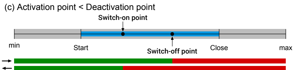
Fig. 51: Hysteresis function
