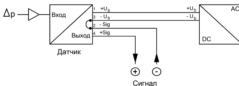
Рис. 4: Трехпроводное подключение с внутренним мостом -U_b / -Sig
