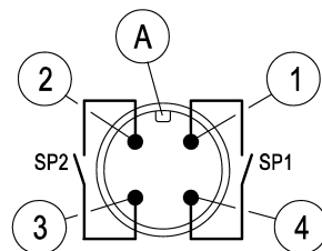
Рис. 17: Электроподключение DE45_LCD
