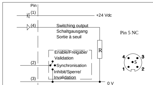
Wiring/Anschlüsse/Raccordement électrique
