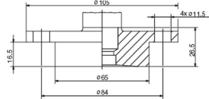
661 зажимной фланец DRD
