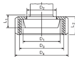
603-607 конический штуцер с накидной гайкой по DIN 11 851
